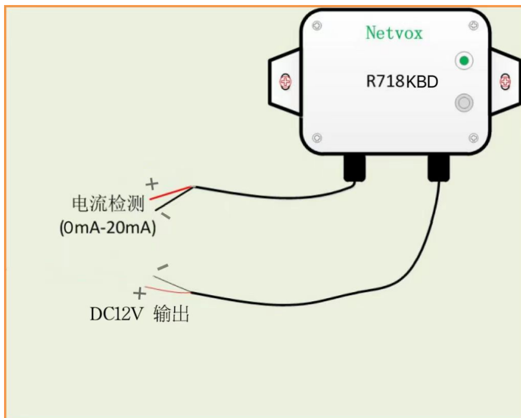
R718KBD 接线示意图
